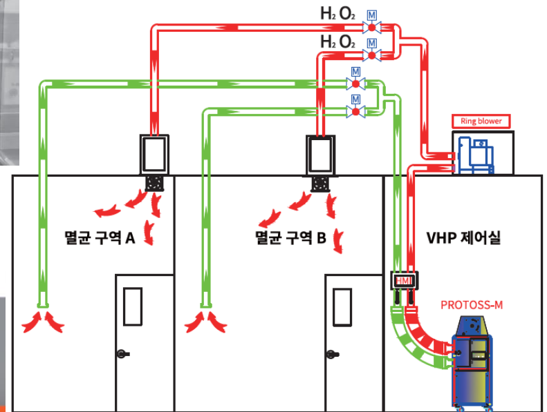
H 2 O 2 멸균 중 배관 계통도
